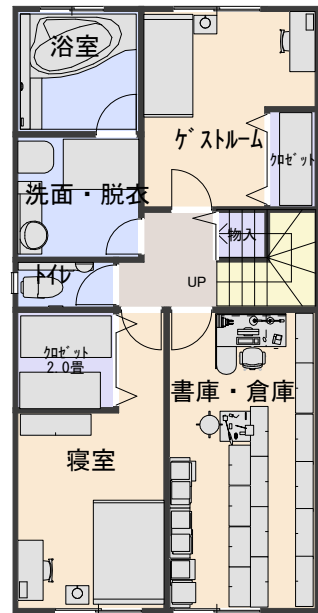
地下平面図
